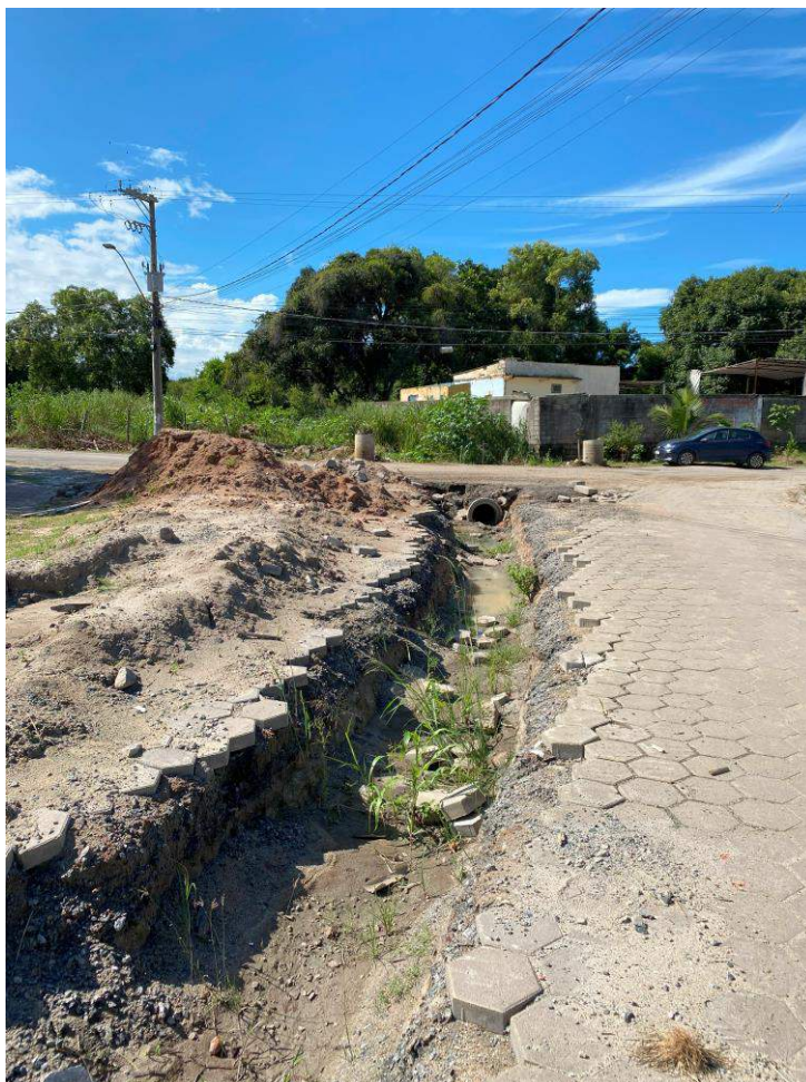
Figura 9-49: Manilha do início da canalização do córrego. Em visita em 2023 aparentava um início de obra no local.
