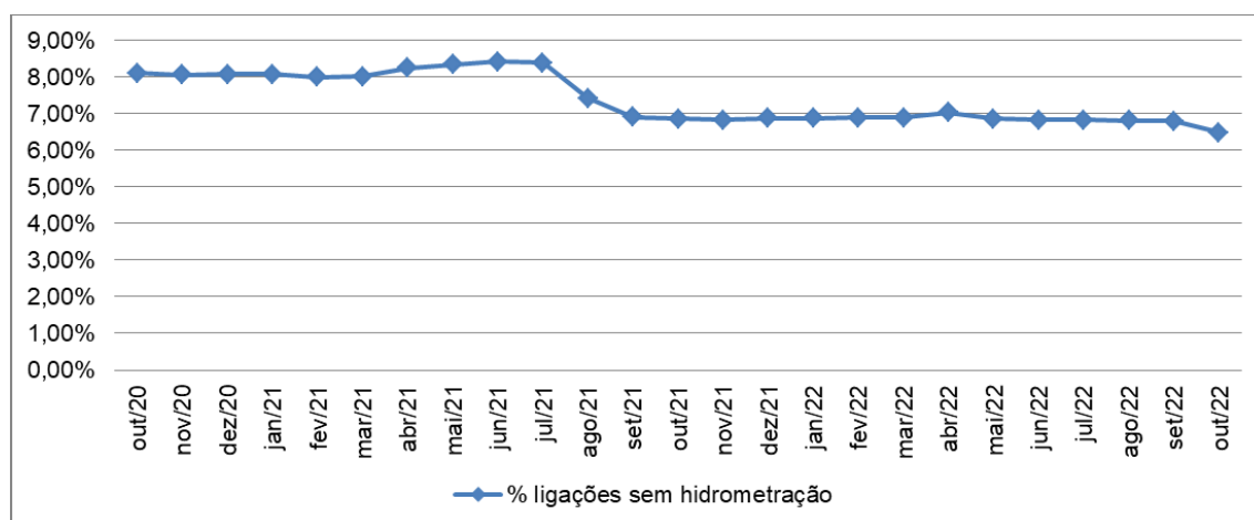
Figura 6-23: Evolução do percentual de ligações sem hidrômetros – SAA SAAE
