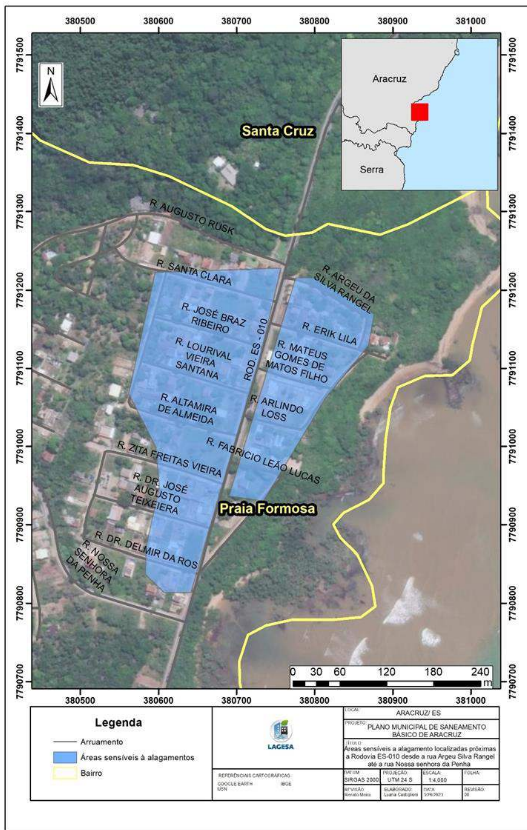
Figura 9-89: Áreas sensíveis a alagamento localizadas próximas a Rodovia ES-010 desde a Rua Argeu Silva Rangel até a Rua Nossa Senhora da Penha.
