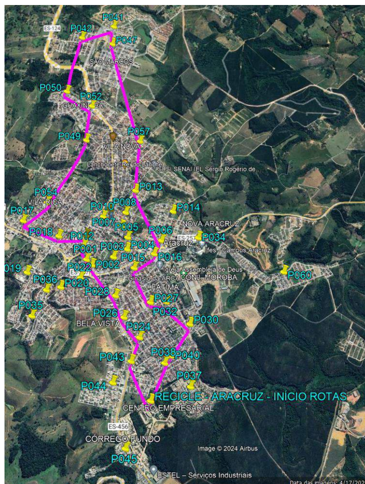
Figura 35-7: Sequência dos pontos a serem atendidos pelo veículo 1 (viagem inicia na Recicle e termina na Recicle)
